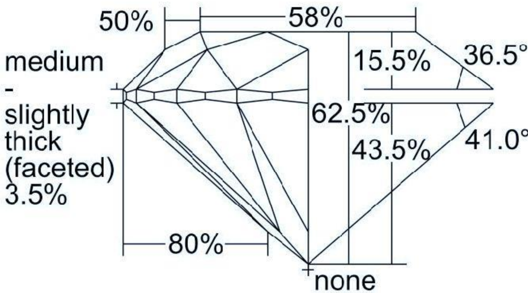
Profile to actual proportions
